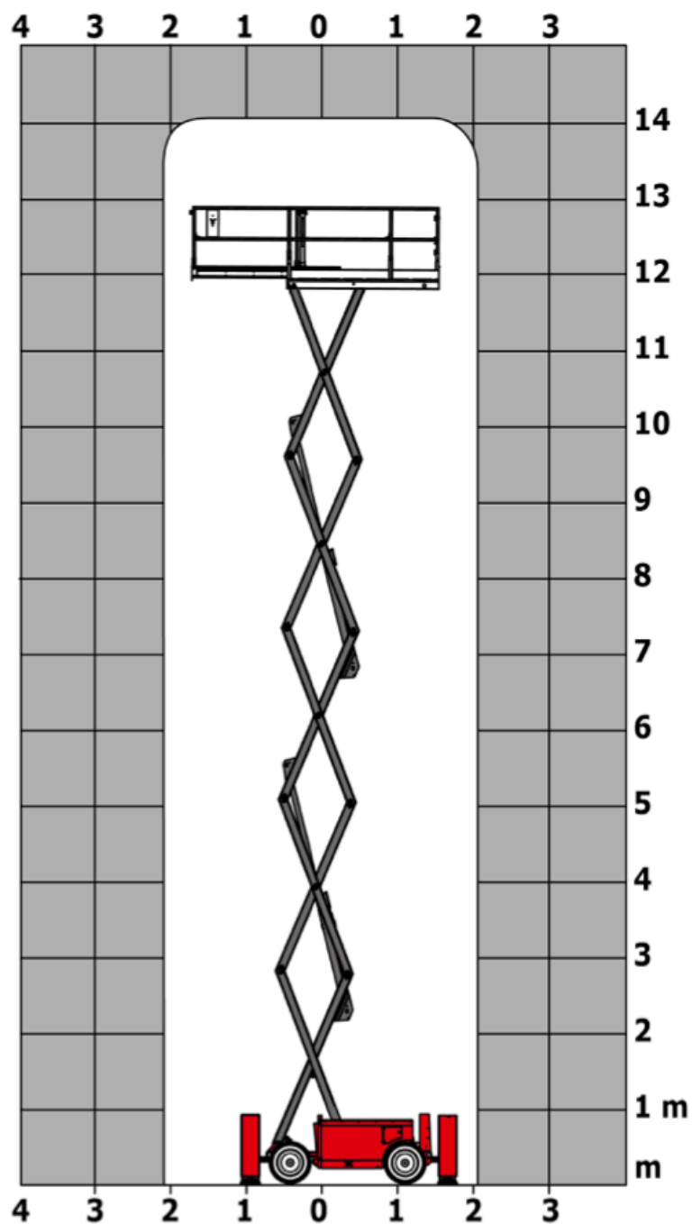
Abaque de charge pour nacelles élévatrices
